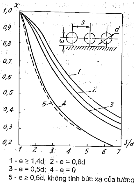
Hình 3-16. Hệ số góc của dàn ống tròn một dãy.
