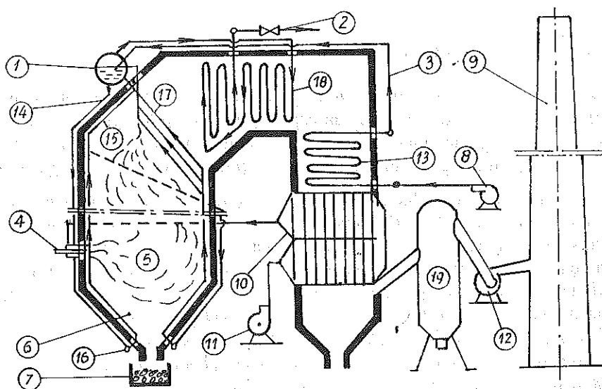
Hình 1-1c. Lò đốt than phun.
