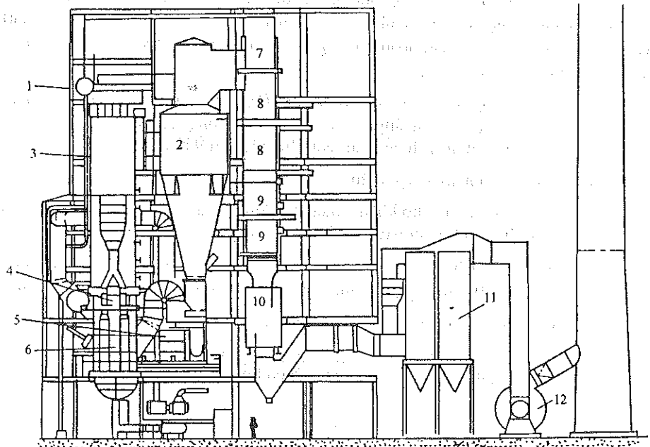
Hình 2-36. Sơ đồ nguyên lý lò hơi tầng lỏng có tái tuần hoàn.
