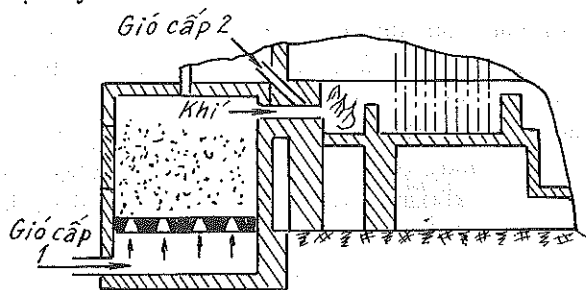
Hình 2-14. Buồng đốt khí hoá.
