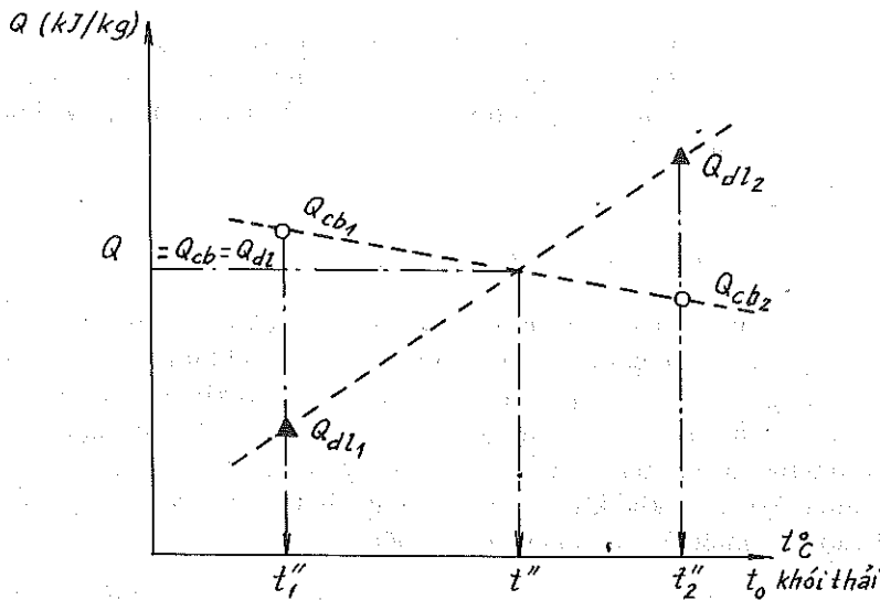
Hình 3-17. Xác định nhiệt độ sản phẩm cháy.
