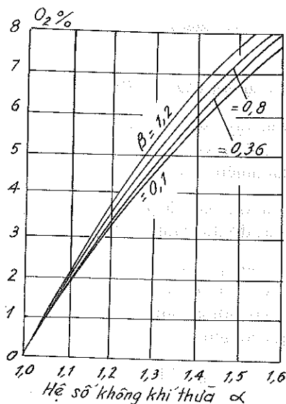
Hình 1-2b. Quan hệ của O_2 với \alpha
