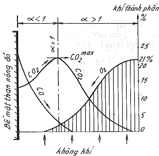
Hình 2-1. Sự phân bố các chất khí xung quanh hạt than.
