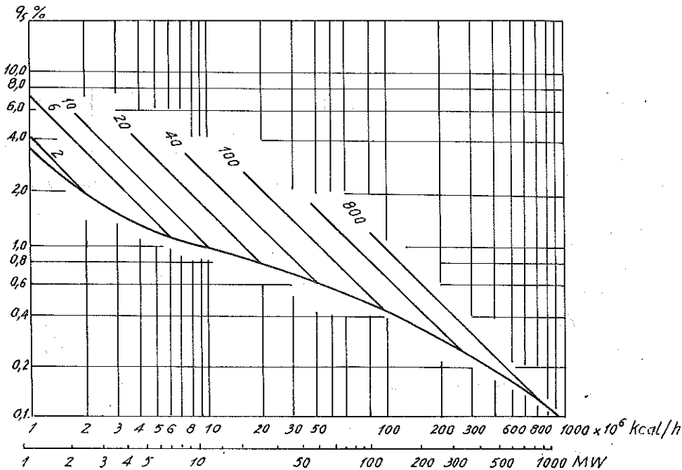
Hình 1-4b. Quan hệ giữa q_s với năng suất nhiệt BQ_1 , \text{kcal/h} hoặc \text{MW} .
