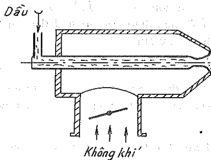
Hình 2-25. Vòi phun dầu bằng không khí.
