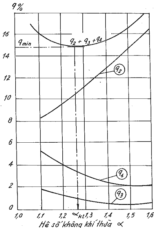
Hình 1-3. Chọn \alpha tối ưu
