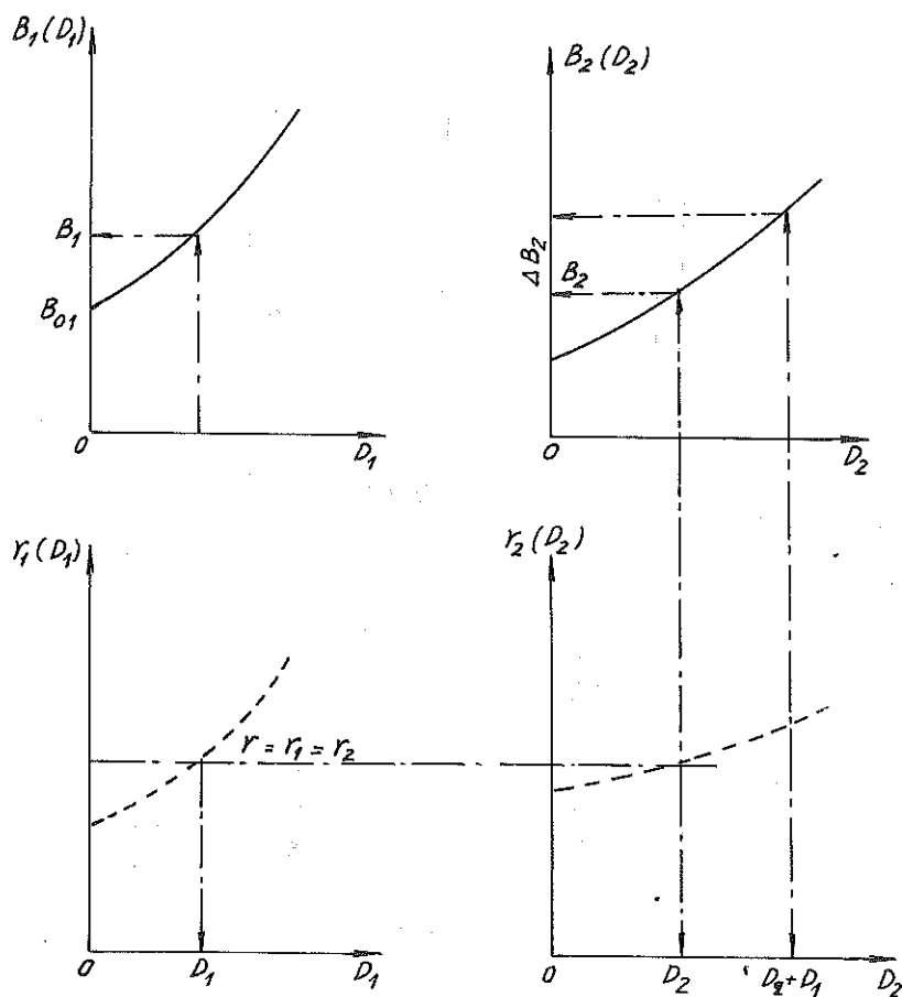
Hình 6-2. Chuyển phụ tải sang một lò.
