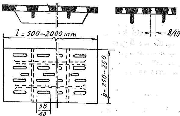
Hình 2-6. Ghi tấm.
