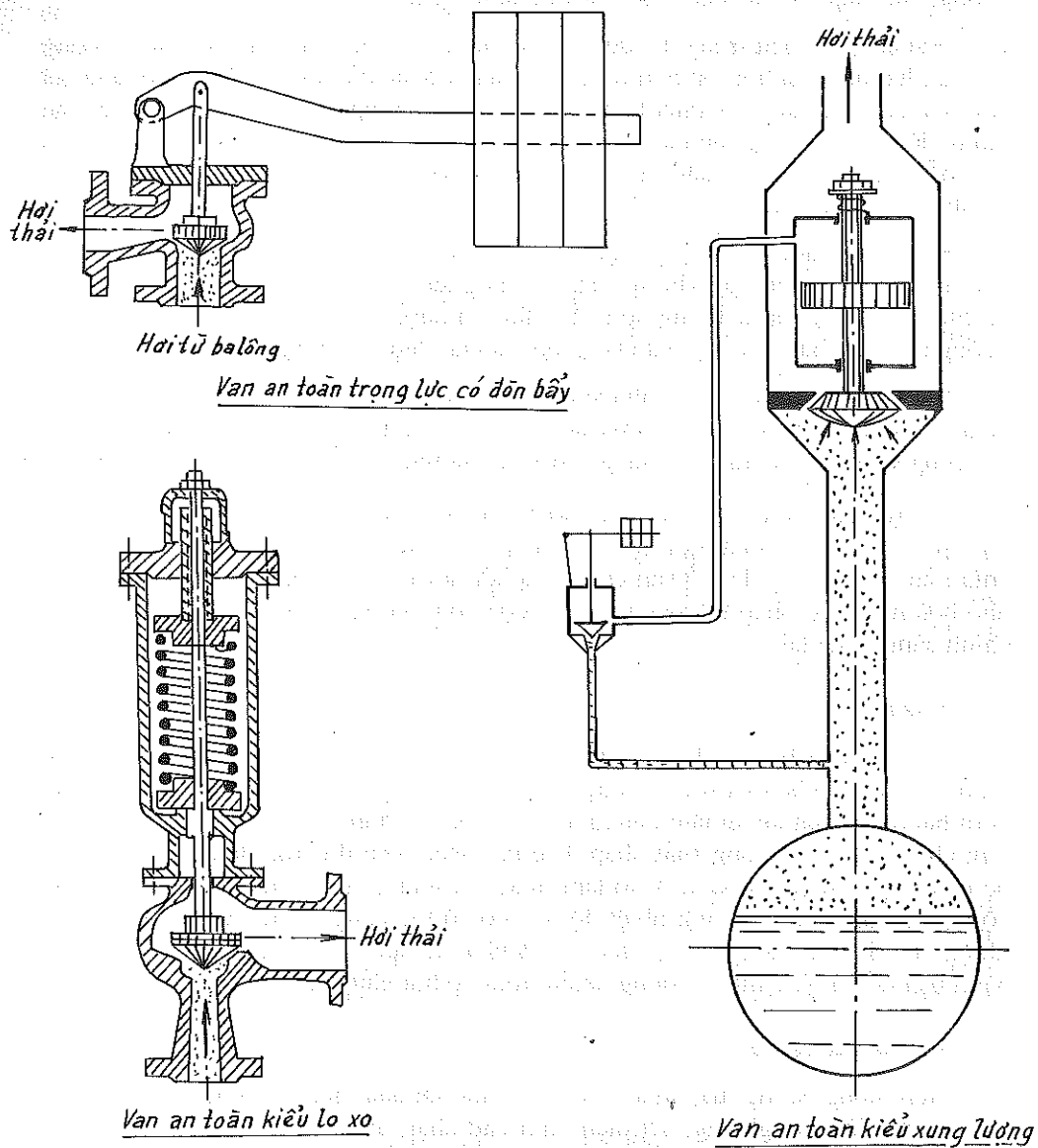
Hình 5-2. Cấu tạo các loại van an toàn.
