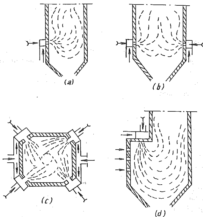
Hình 2-22. Cách bố trí vòi phun trong buồng lửa.
