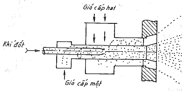
Hình 2-31. Vòi phun đốt ngọn lửa không sáng.
