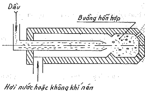
Hình 2-24. Vòi phun dầu có áp suất cao.
