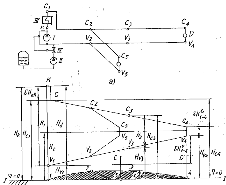
Hình 7-5. Đồ thị đo áp của mạng nước hai đường ống.
