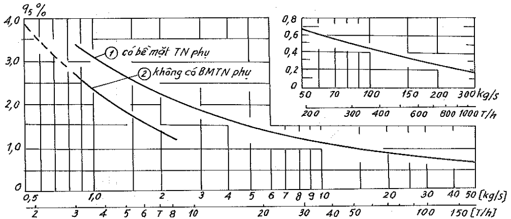
Hình 1-4a. Quan hệ giữa q_5 với sản lượng hơi D , kg/s hoặc T/h .
