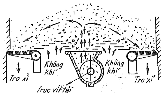
Hình 2-11. Buồng lửa cấp than bằng vít tải.
