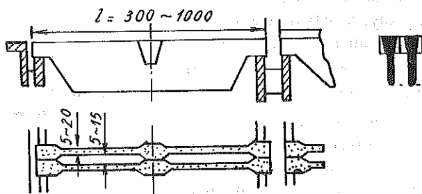
Hình 2-7. Ghi thanh.
