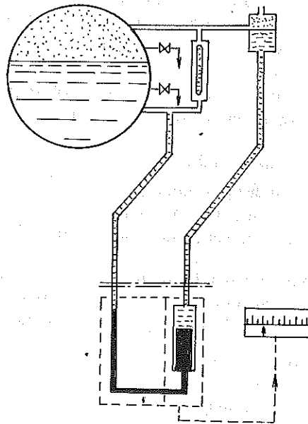
Hình 5-1. Ống thuỷ đo mức lỏng.
