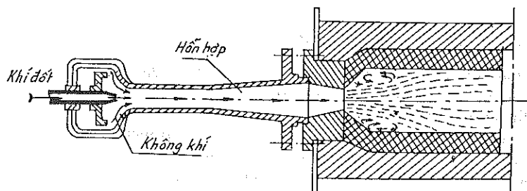
Hình 2-32. Vòi phun không có ngọn lửa.
