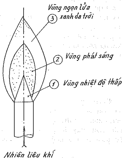
Hình 2-27. Ngọn lửa sáng.
