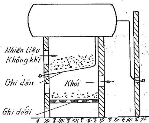
Hình 2-13. Buồng đốt ghi kép.
