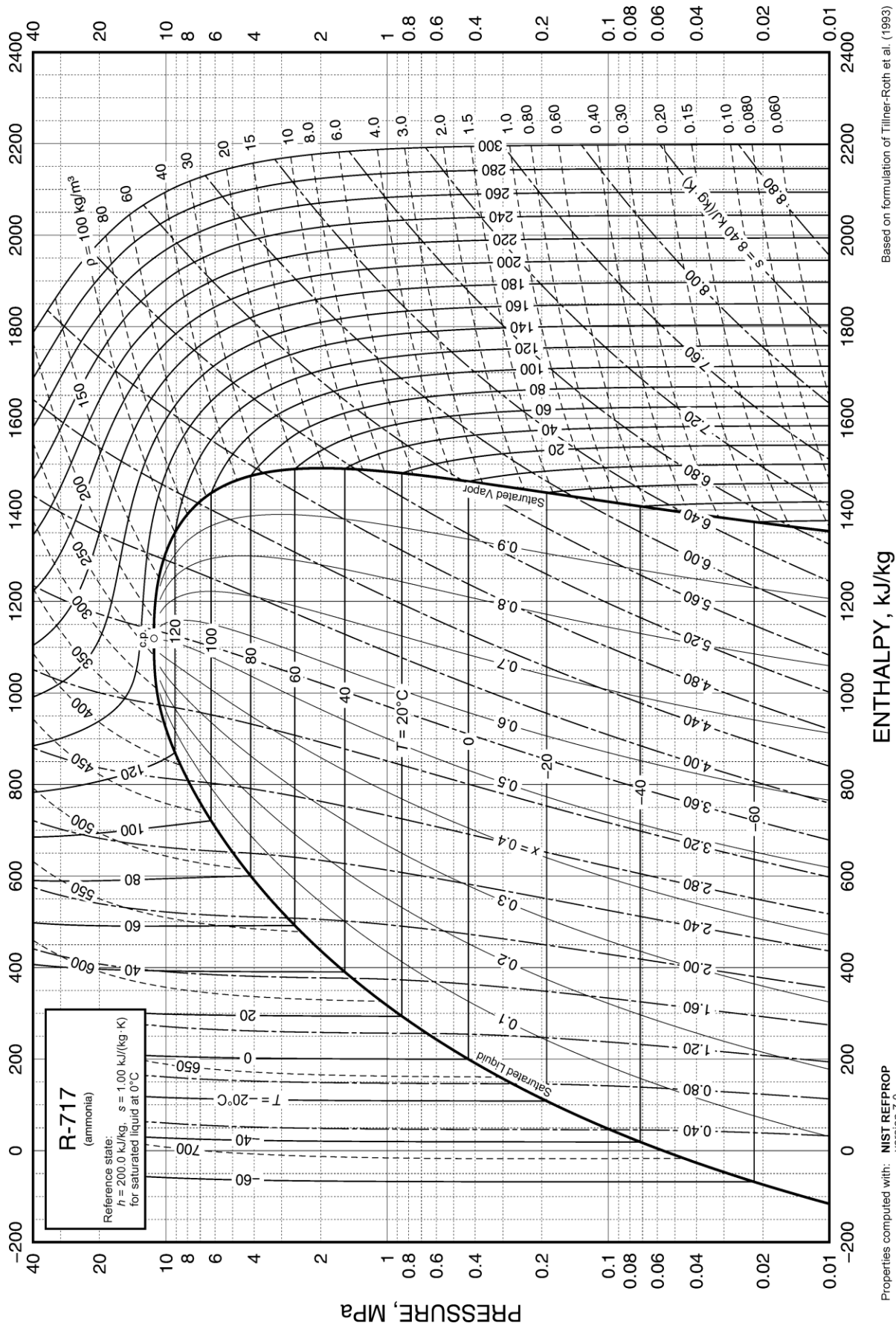
PHỤ LỤC 6: ĐỒ THỊ MÔI CHẤT R717 (Ammonia)
